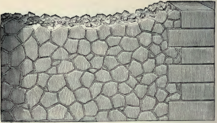
Opus incertum.
